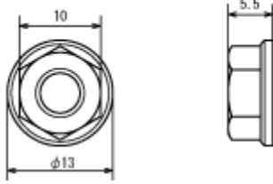
M6 Flange Nut
