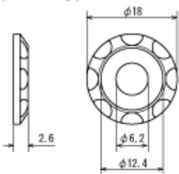
Spacer type01 (mm)
