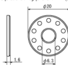
Spacer type31 (mm)
