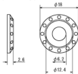
Spacer type02 (mm)
